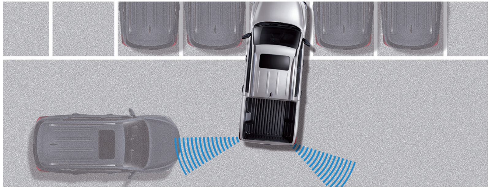
4 RCTW 後方車側警示系統 停車時，透過攝影機即時呈現後方視野，加上雷達偵測後方死角，同步於兩側後視鏡警示提醒，避免意外。
